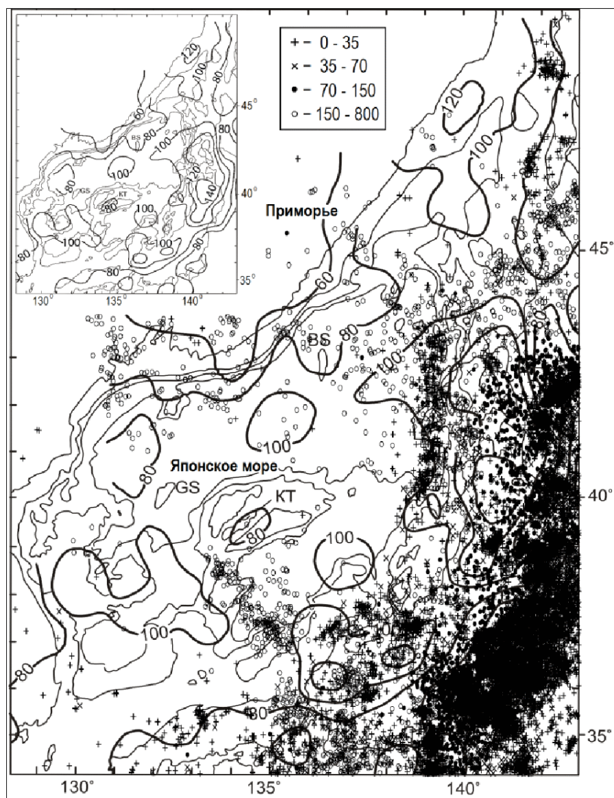
Рис. 4. Контурная карта теплового потока Японского моря [17] с эпицентрами землетрясений [19] и линейменами. Контурсы проведены через 20 мВт/м 2
