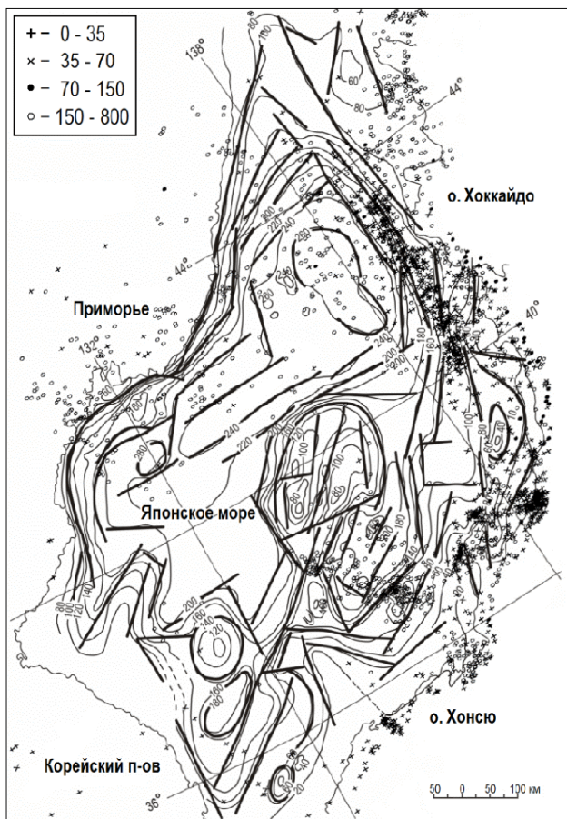
Рис. 2. Схематическая карта гравитационных аномалий в редукции Буге (изолинии – в мГал) Японского моря [15] с эпицентрами землетрясений [19] и линейными зонами градиентов
