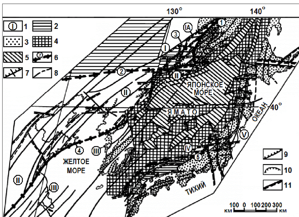
Рис. 1. Схема тектонического районирования Японского звена Западно-Тихоокеанской зоны перехода континент – океан (по: [4] с изменениями):
