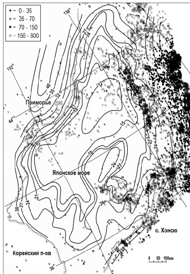
Рис. 3. Карта рельефа поверхности Мохоровичича Япономорской зоны (изолинии – в км) [9] с эпицентрами землетрясений [19] и линеаменами
