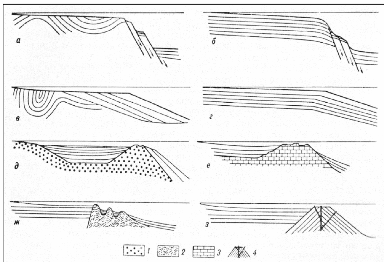
Рис. 1 а–з. Модели континентальных шельфов [14]:
